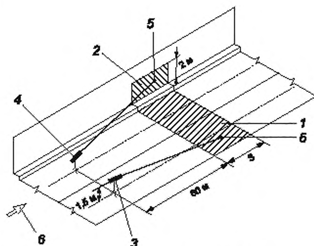
Рисунок Д.3 — Расположение контрольных точек на стене тоннеля
