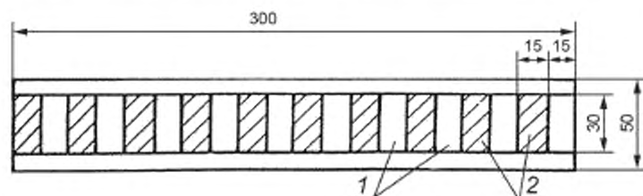
Рисунок В.1 — Схема шкалы набора образцов
