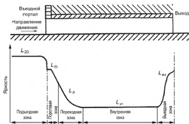
Рисунок Д.1 — Яркостные зоны тоннеля
